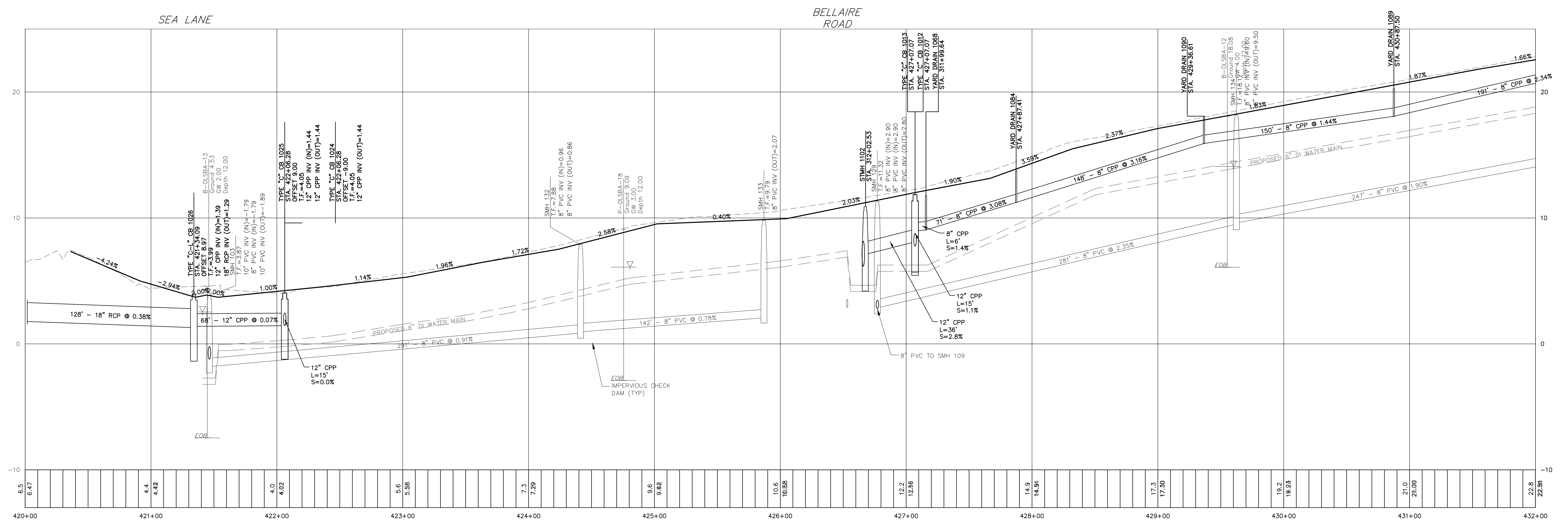
PROFILE STA 420+00 - 432+00 SCALE: H:1"=20' V:1"=2'
