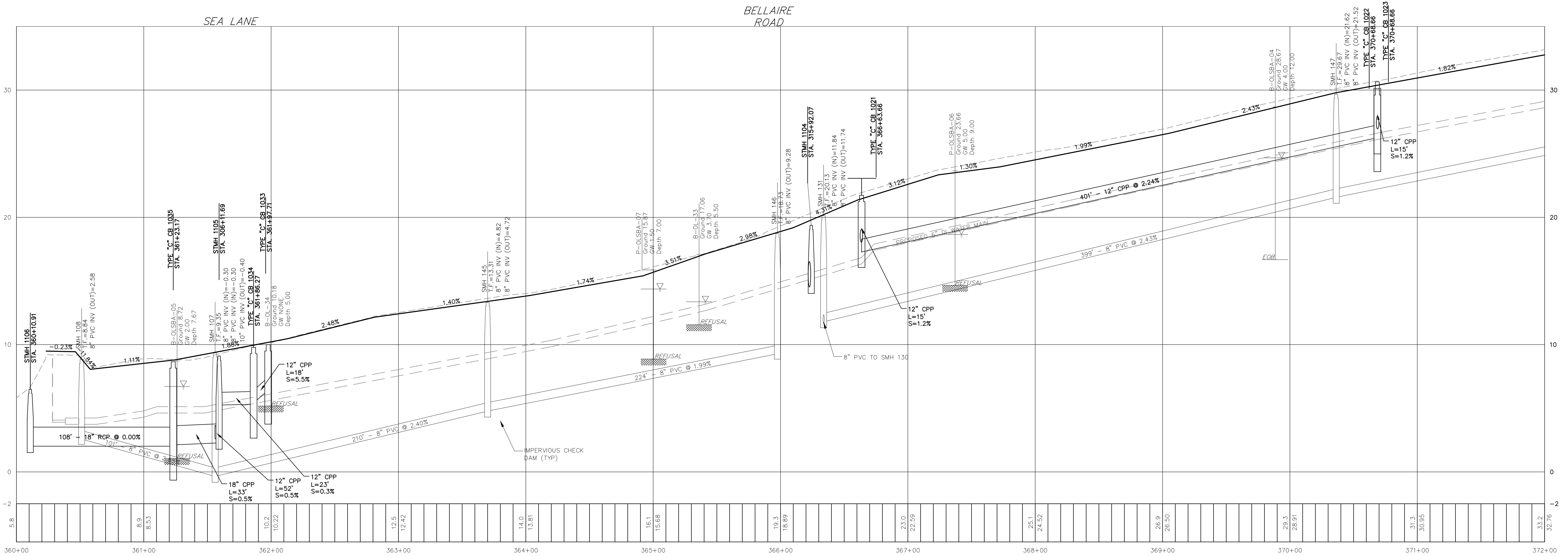
PROFILE STA 360+00 - 372+00 SCALE: H: 1"=20' V: 1"=2'
