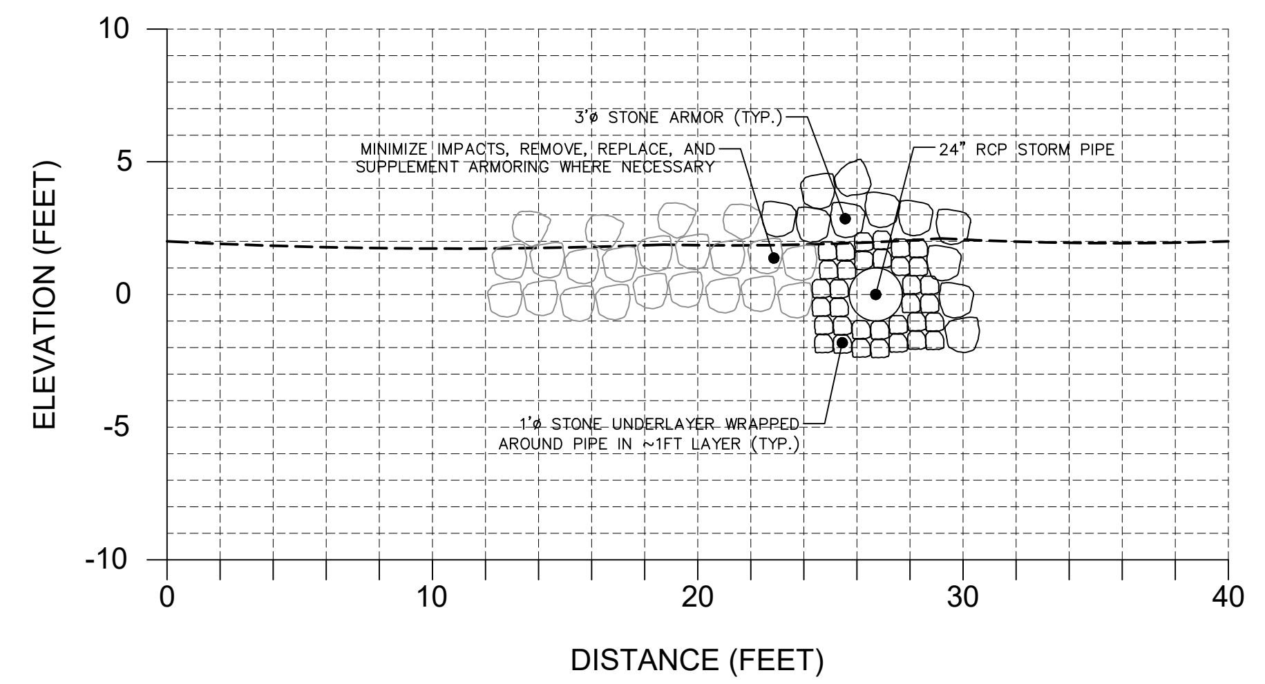
A OLSBA JETTY OUTFALL SCALE: N.T.S.
