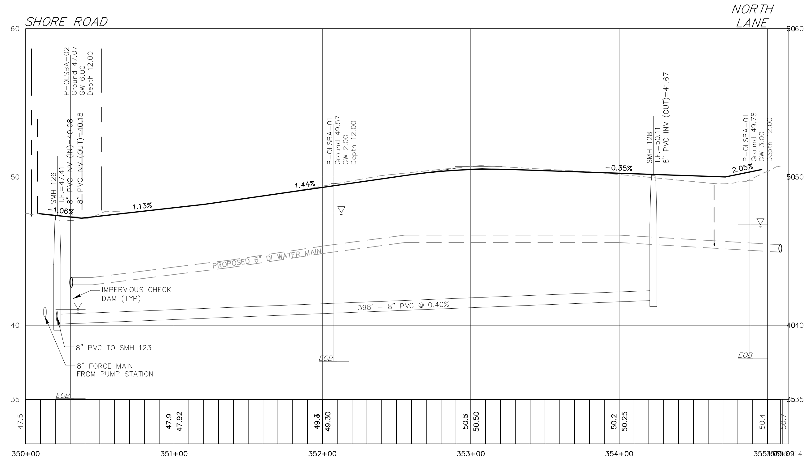
PROFILE STA 350+00 - 355+14 SCALE: H: 1" = 20' V: 1" = 2'
