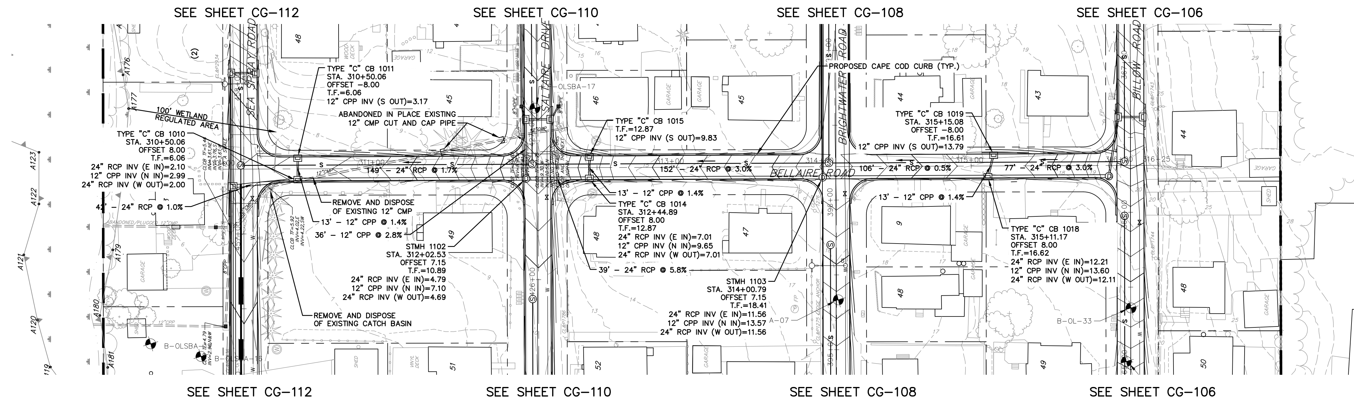
PLAN STA. 310+00 - 316+25 SCALE: H: 1" = 40'
