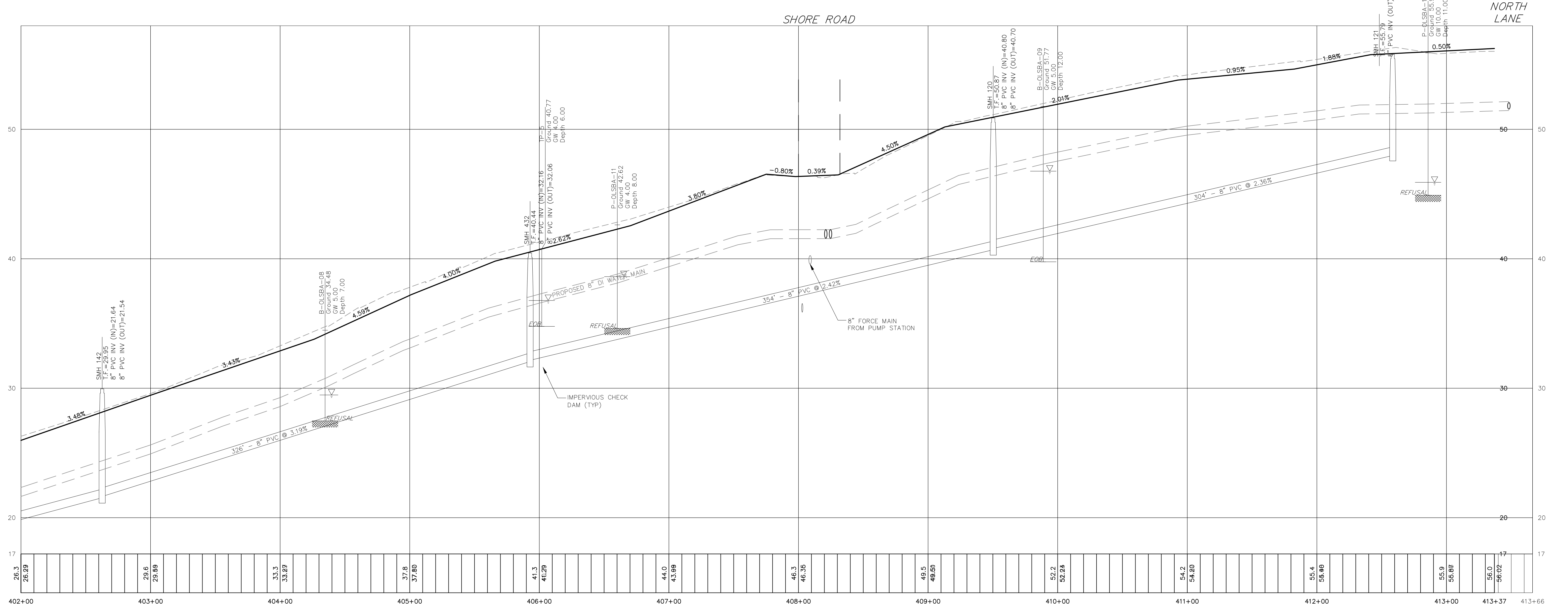
PROFILE STA 402+00 - 413+66 SCALE: H: 1"=20' V: 1"=2'
