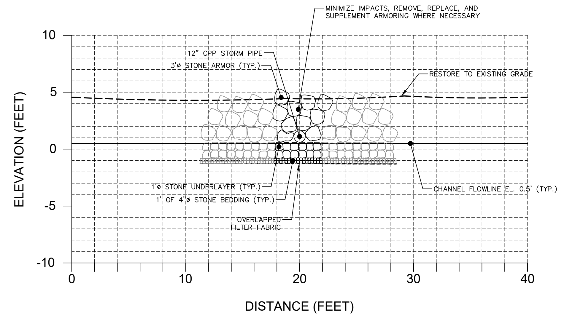
B SHEFFIELD BROOK OUTFALL SCALE: N.T.S.
